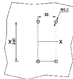
Шаблон для разметки монтажной панели
