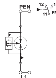
Электрическая схема
